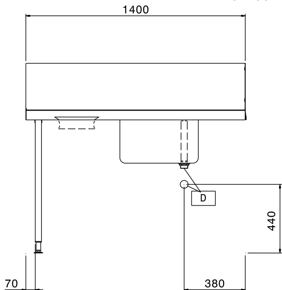
Front aanzicht
