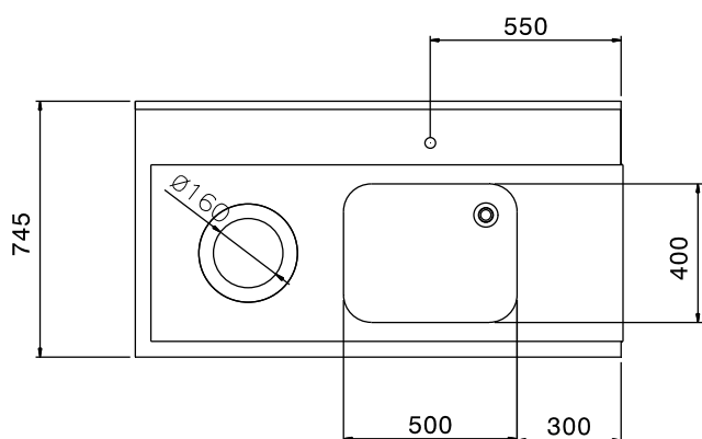
Boven aanzicht
